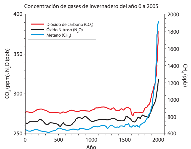
Figura 1: Concentración atmosférica del dióxido de carbono, metano y óxido nitroso durante los pasados 2005 años. Estos son gases de invernadero que ocurren naturalmente. Datos obtenidos en testigos de hielo y mediciones contemporáneas 4 .
